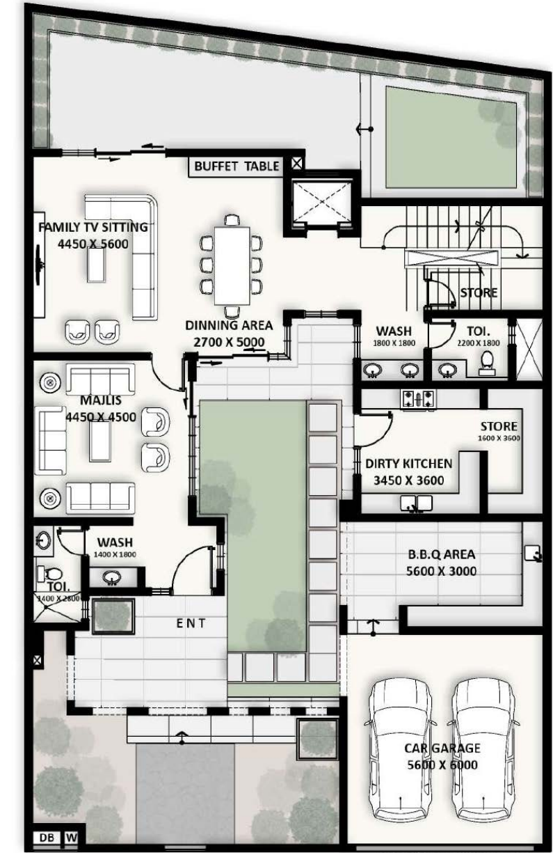
الطابق الأرضي
