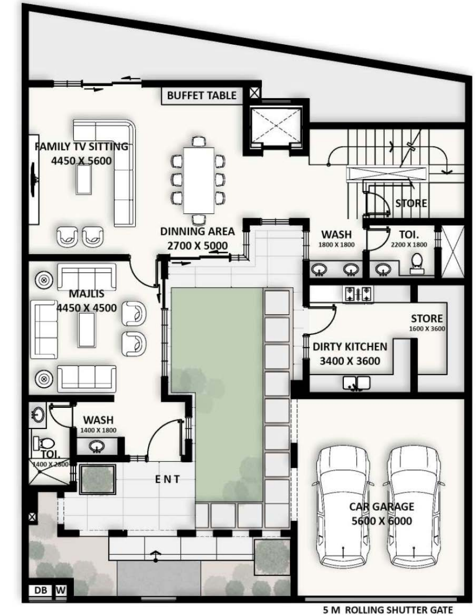
الطابق الأرضي
