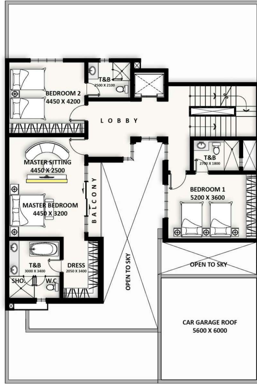
الطابق الأول
