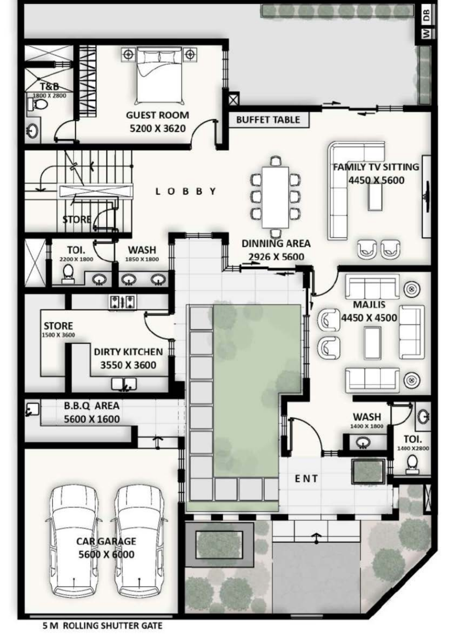
الطابق الأرضي
