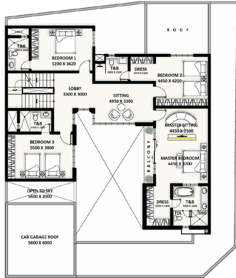
الطابق الأول
