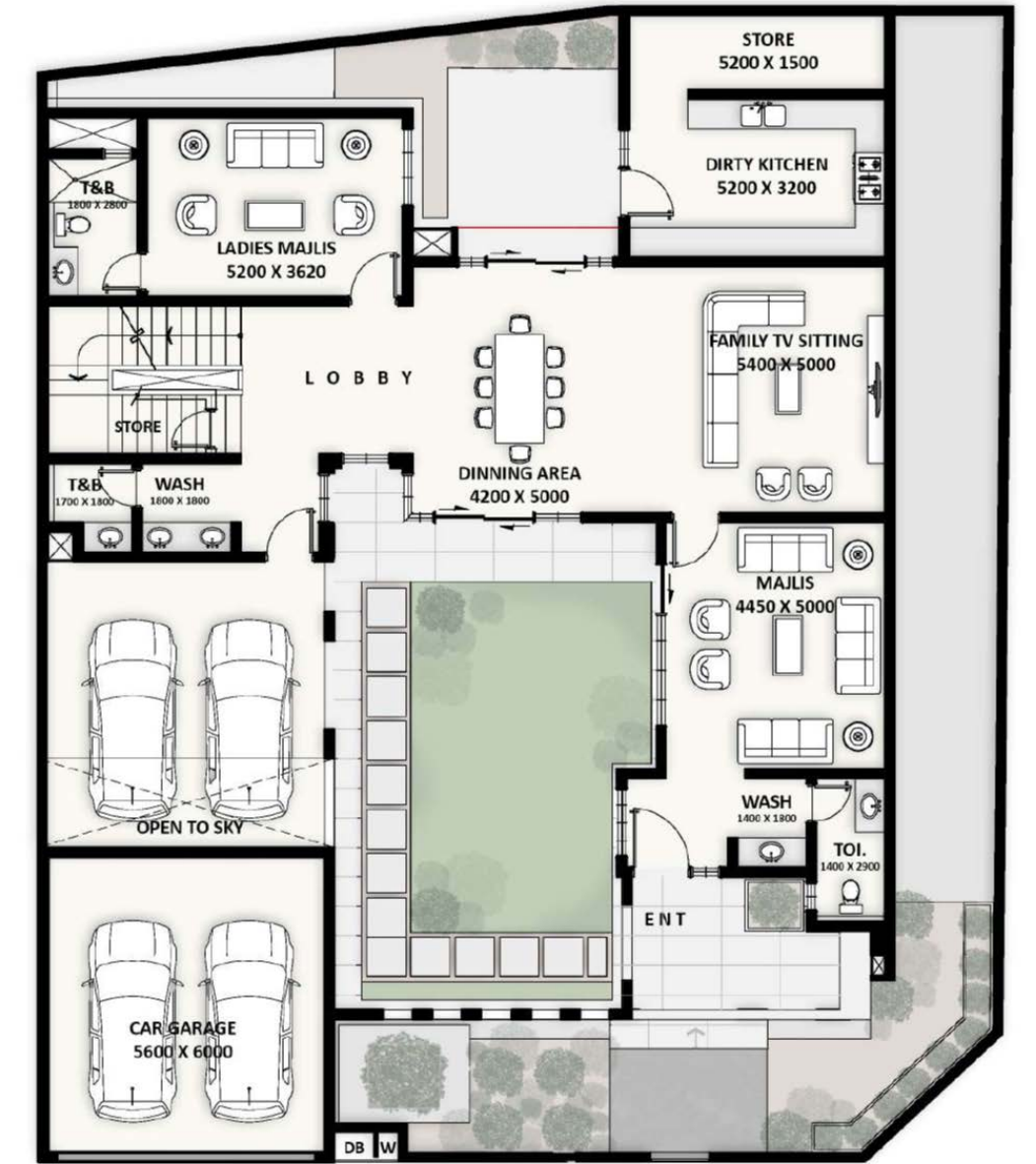
الطابق الأرضي
