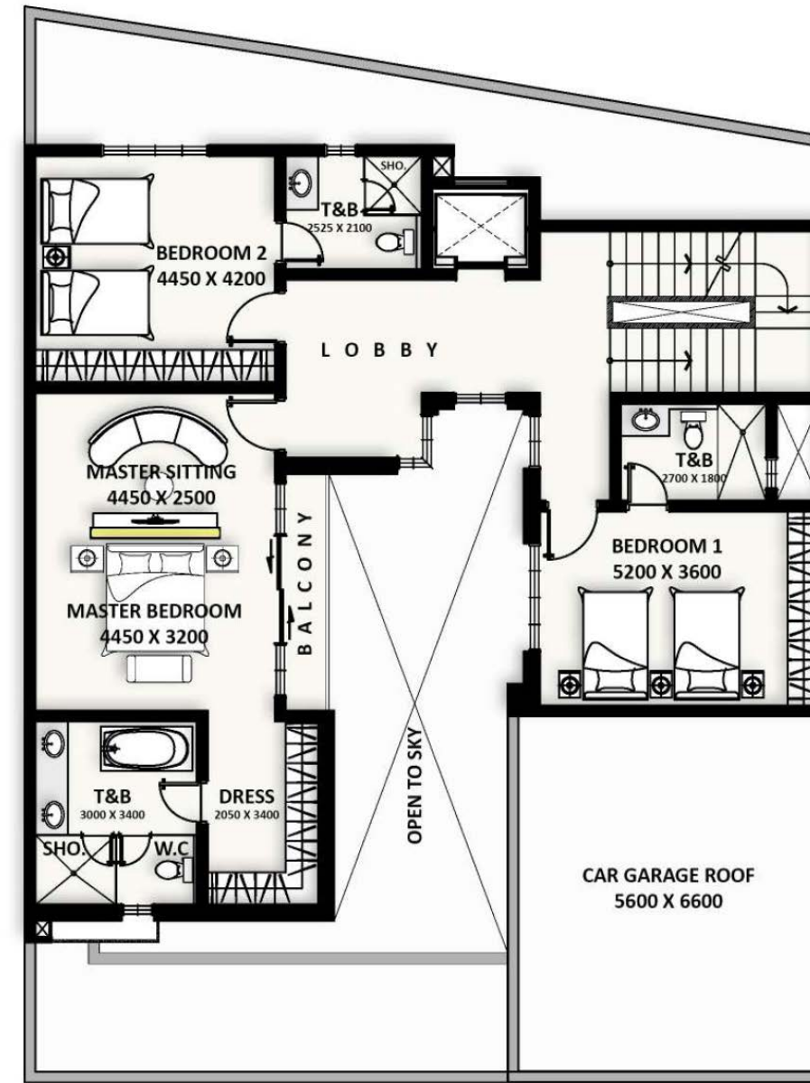
الطابق الأول
