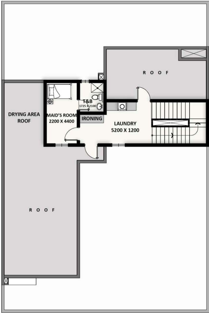
السطح
