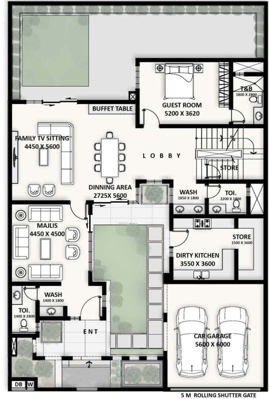
الطابق الأرضي
