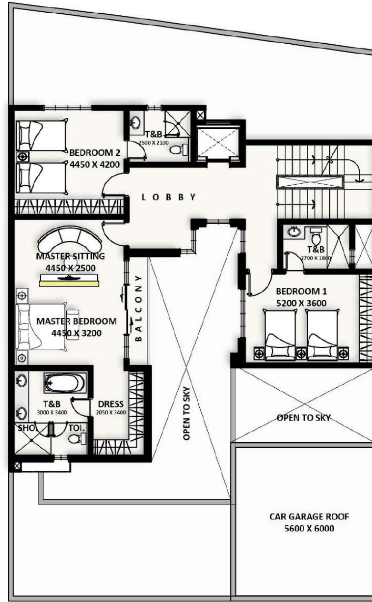
الطابق الأول
