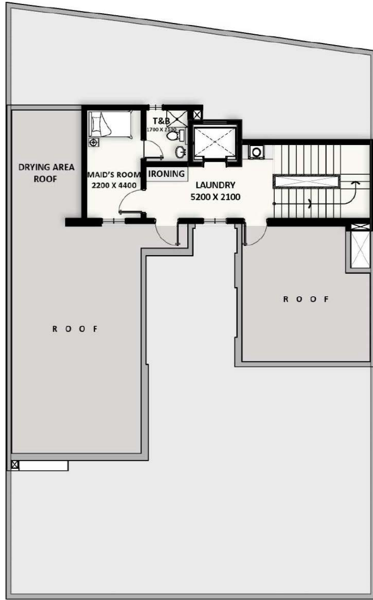
السطح
