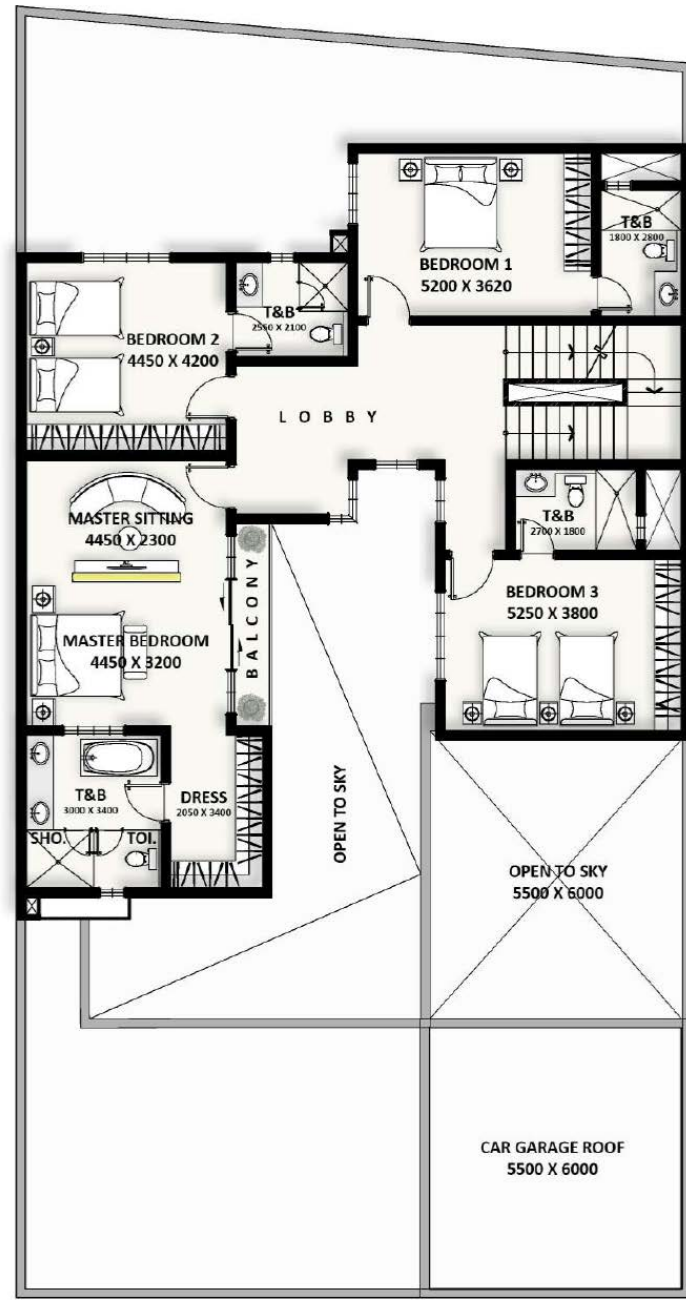
الطابق الأول
