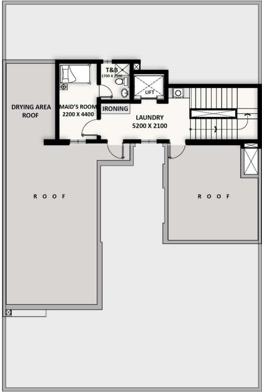
السطح
