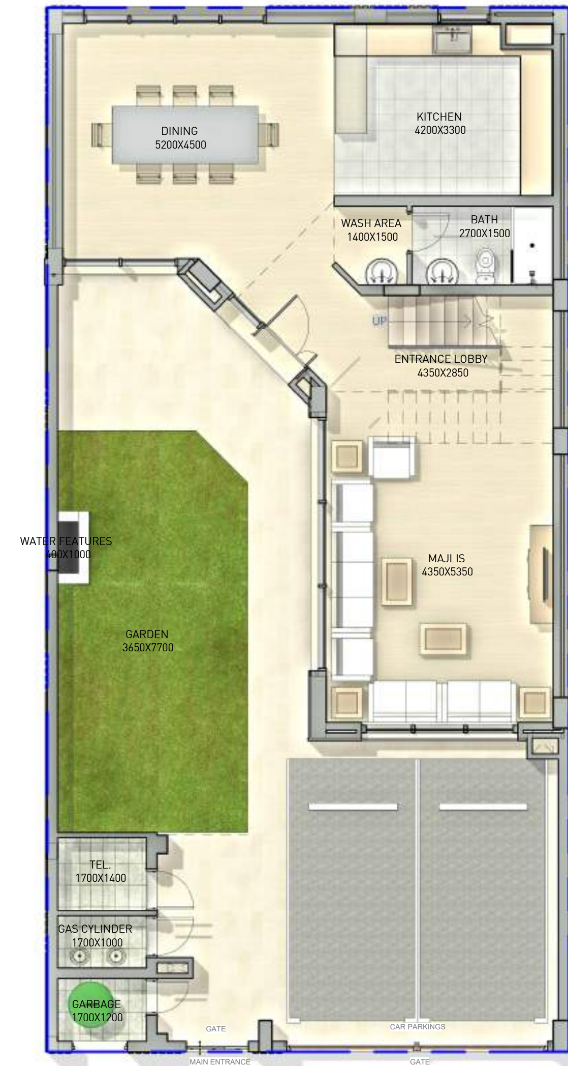
الطابق الأرضي
