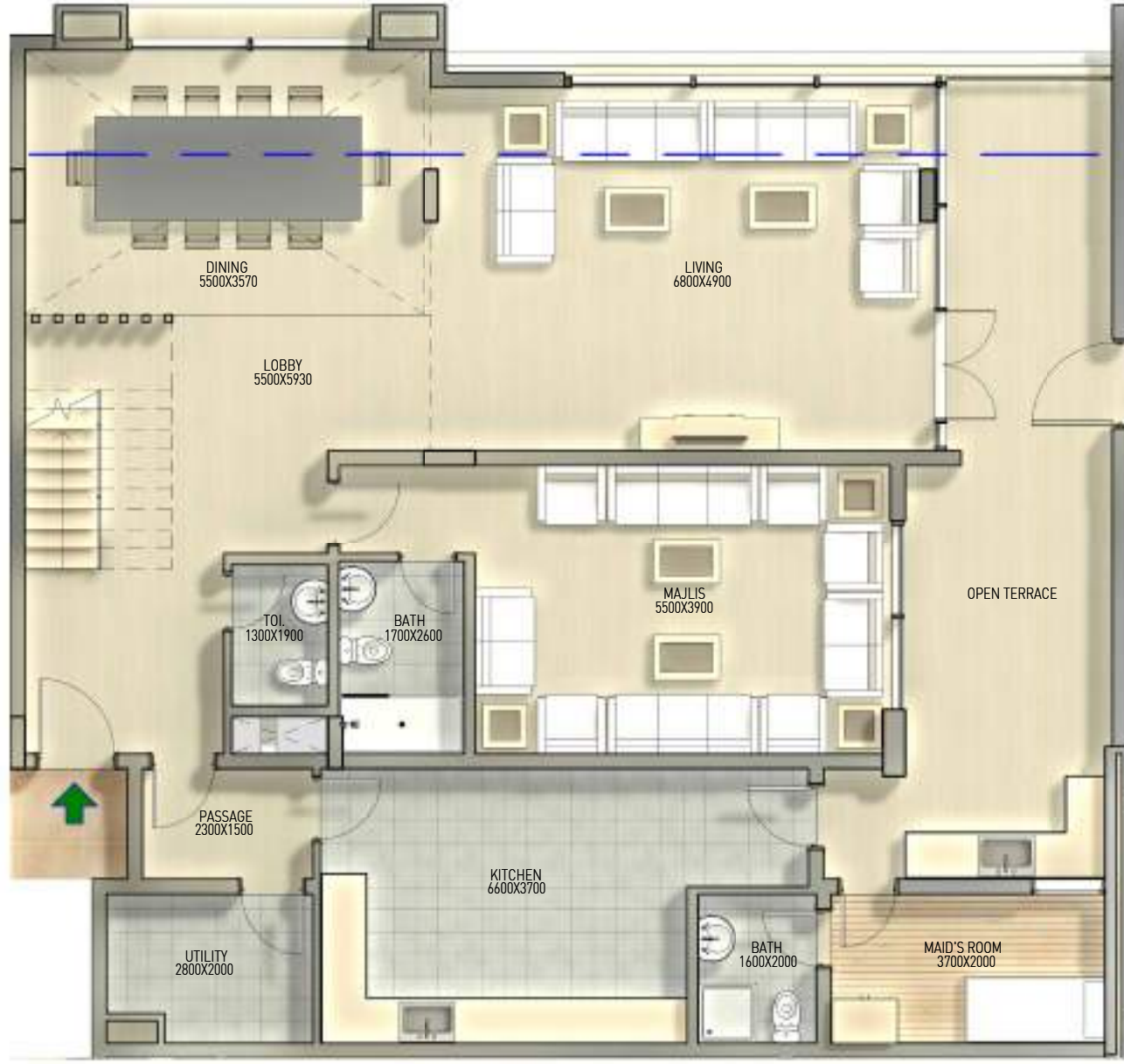
الطابق الأول
